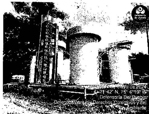
Imagen 8. Planta de tratamiento de lixiviados
