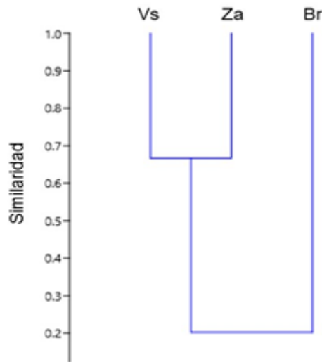
Figura 90. Análisis de diversidad beta para reptiles por hábitat.
