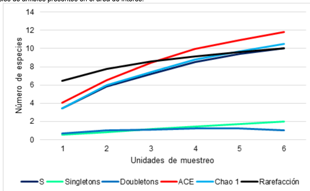
Figura 86. Curva de acumulación de especies de anfibios.
