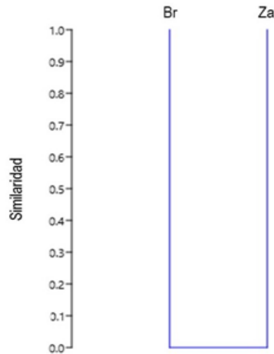
Figura 87. Análisis de diversidad beta para anfibios por cobertura. Fuente: Elaboración Propia
