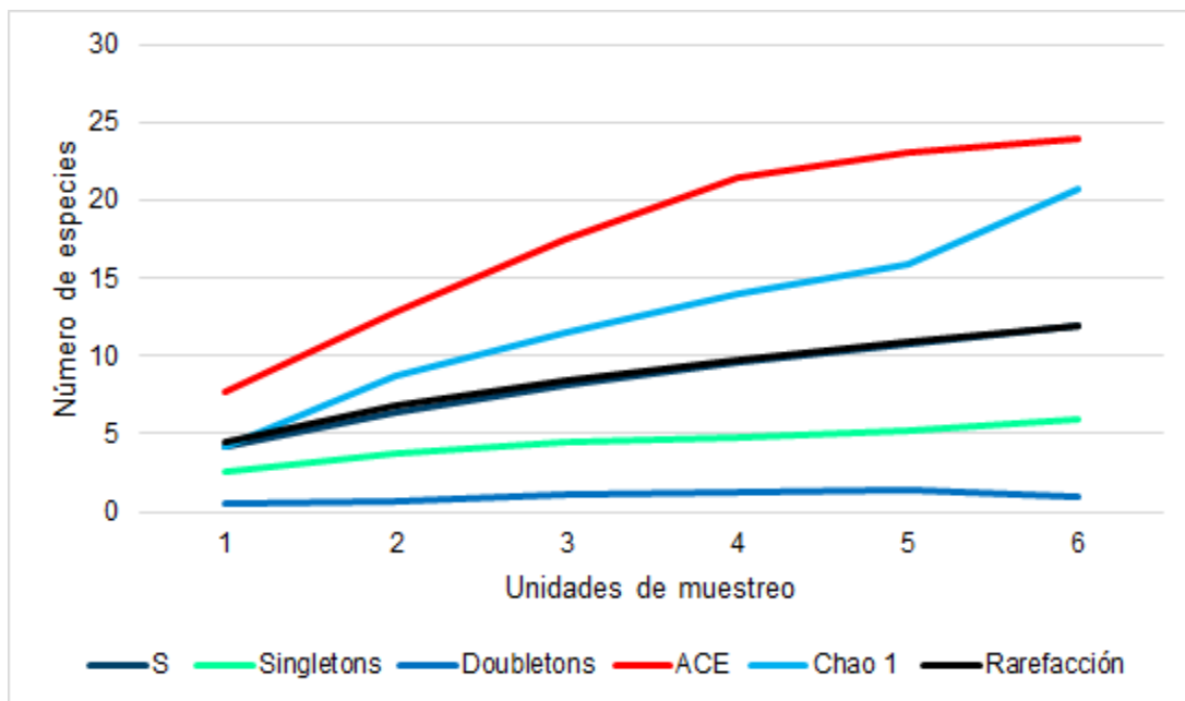
Figura 89. Curva de acumulación de especies de reptiles para el área de influencia.
