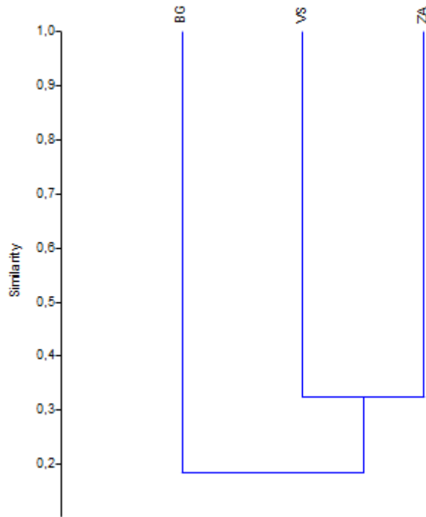
Figura 84. Cluster de similaridad Bray-Curtis entre los hábitats con presencia de aves en el AIB del proyecto. Fuente: Elaboración Propia
