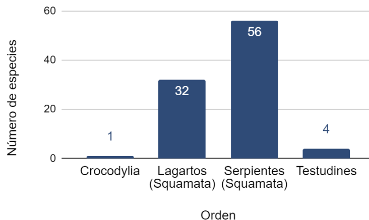
Figura 74. Riqueza de especies para los tres órdenes de reptiles asociados a la región del proyecto.
