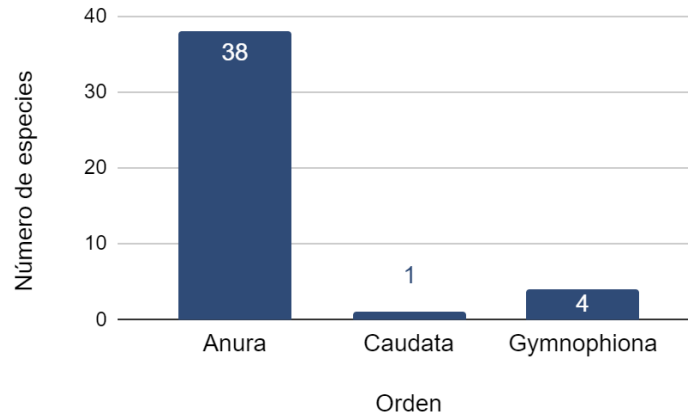
Figura 72. Riqueza de especies por orden de anfibios asociados a la región del proyecto Fuente: Elaboración Propia
