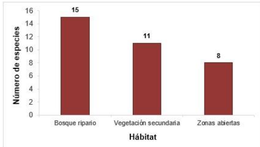
Figura 97. Asociación de las especies de mamíferos con el hábitat en el área de influencia biótica del Proyecto Fuente: Elaboración Propia
