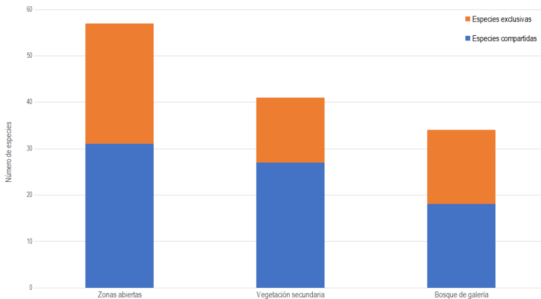
Figura 85. Número de especies por tipo de hábitat para las aves del AIB del proyecto Fuente: Elaboración Propia
