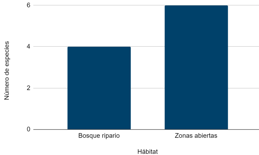
Figura 88. Riqueza de anfibios por hábitat en el área de influencia. Fuente: Elaboración Propia
