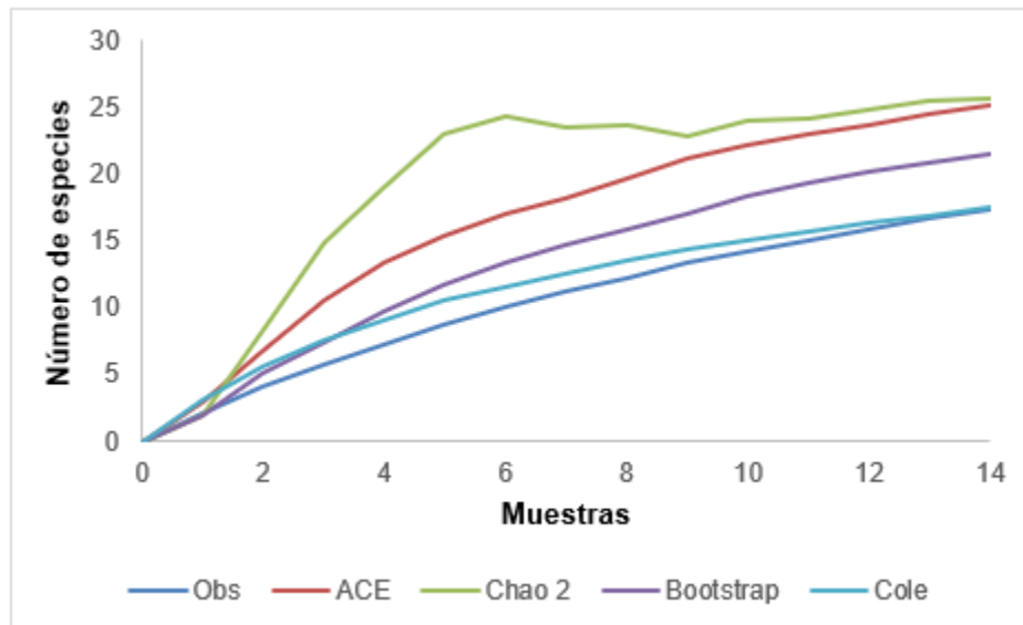
Figura 92. Curva de acumulación de especies de mamíferos del área de influencia biótica del Proyecto Fuente: Elaboración Propia
