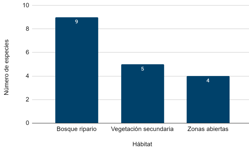
Figura 91. Riqueza de reptiles por hábitat. Fuente: Elaboración Propia
