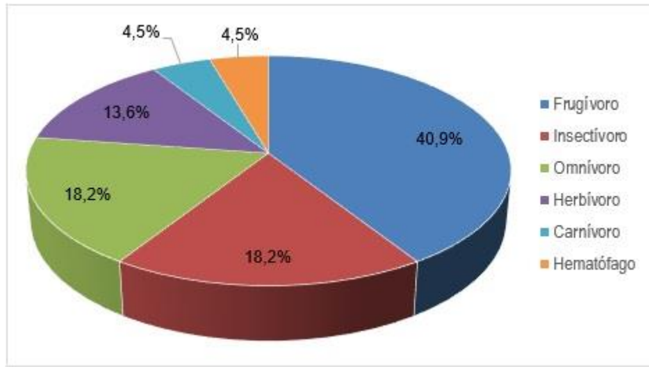
Figura 96. Riqueza de especies de mamíferos por gremio trófico para el área de influencia del Proyecto Fuente: Elaboración Propia
