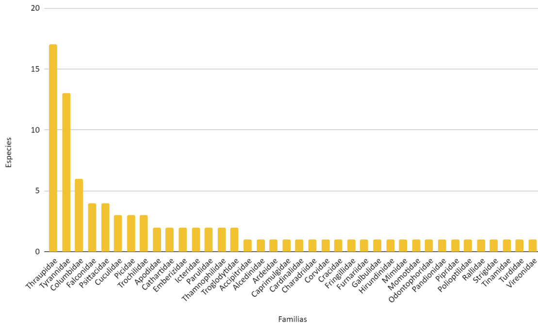
Figura 82. Riqueza de especies para las familias de aves en el AIB del proyecto Fuente: Elaboración Propia
