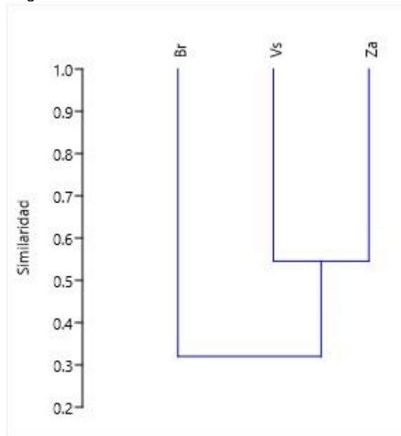
Figura 95. Cluster de similitud Bray-Curtis entre los hábitats con presencia de mamíferos en el área de influencia del Proyecto
