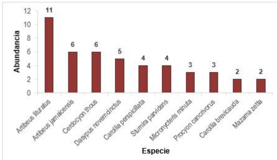
Figura 94. Especies de mamíferos que presentaron la mayor abundancia en el área de influencia biótica del Proyecto Mina La Esmeralda -Título 6823-
