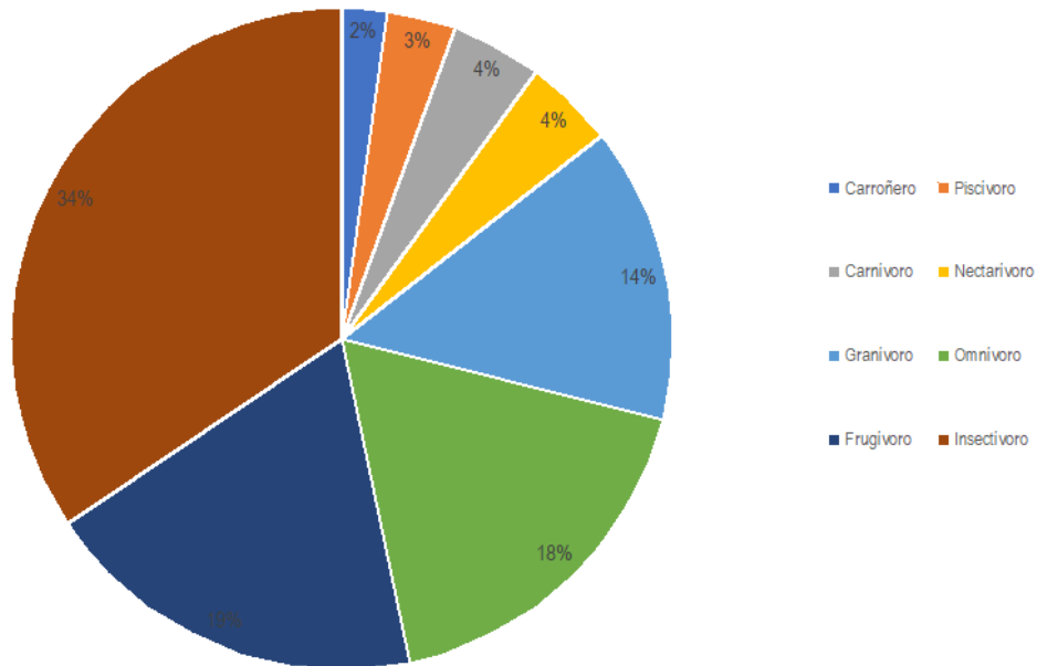
Fotografía 32. Distribución porcentual de especies de aves por gremio trófico para el AIB del proyecto Fuente: Elaboración Propia
