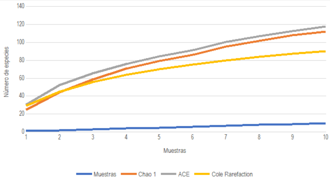
Figura 80. Curva de acumulación de especies de aves del AIB del Proyecto Fuente: Elaboración Propia
