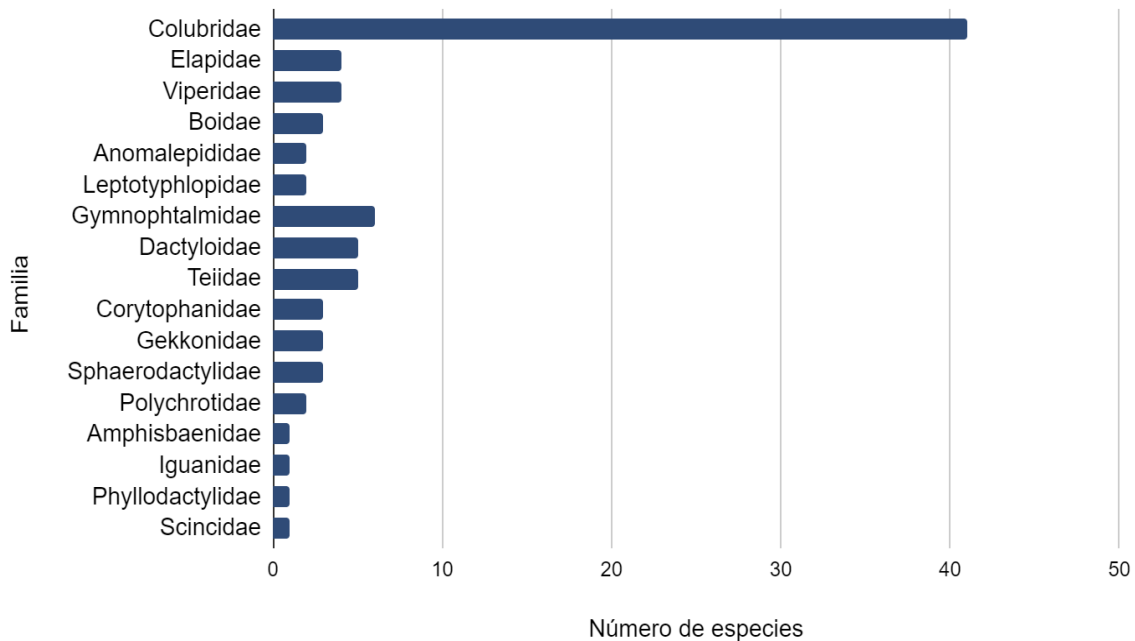
Figura 75. Riqueza de especies por familias de Squamata (Serpientes y lagartos). Fuente: Elaboración Propia
