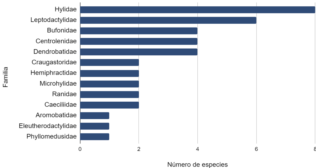
Figura 73. Riqueza de especies por familias de anuros asociadas a la región del proyecto. Fuente: Elaboración Propia
