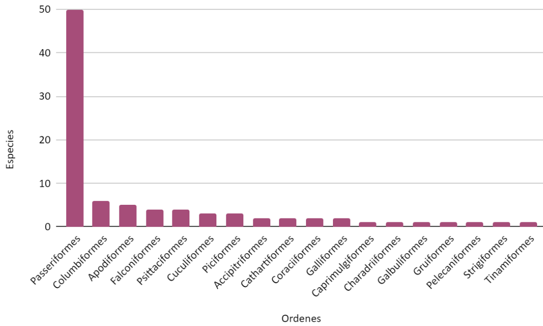
Figura 81. Riqueza de especies para los órdenes de aves en el AIB del proyecto Fuente: Elaboración Propia
