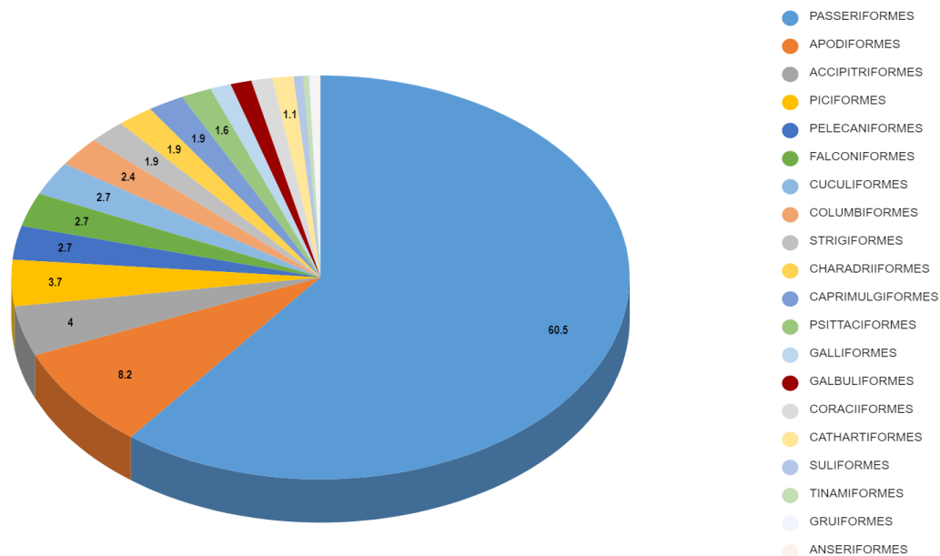
Figura 76. Porcentaje de riqueza por orden para las aves de probable presencia en el contexto regional del proyecto mina la Esmeralda -Título 6823- Fuente: Elaboración Propia
