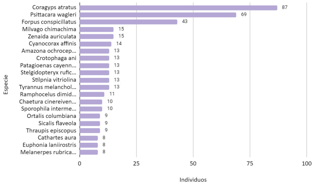
Figura 83. Abundancia de las especies de aves con mayor número de individuos en el AIB Fuente: Elaboración Propia
