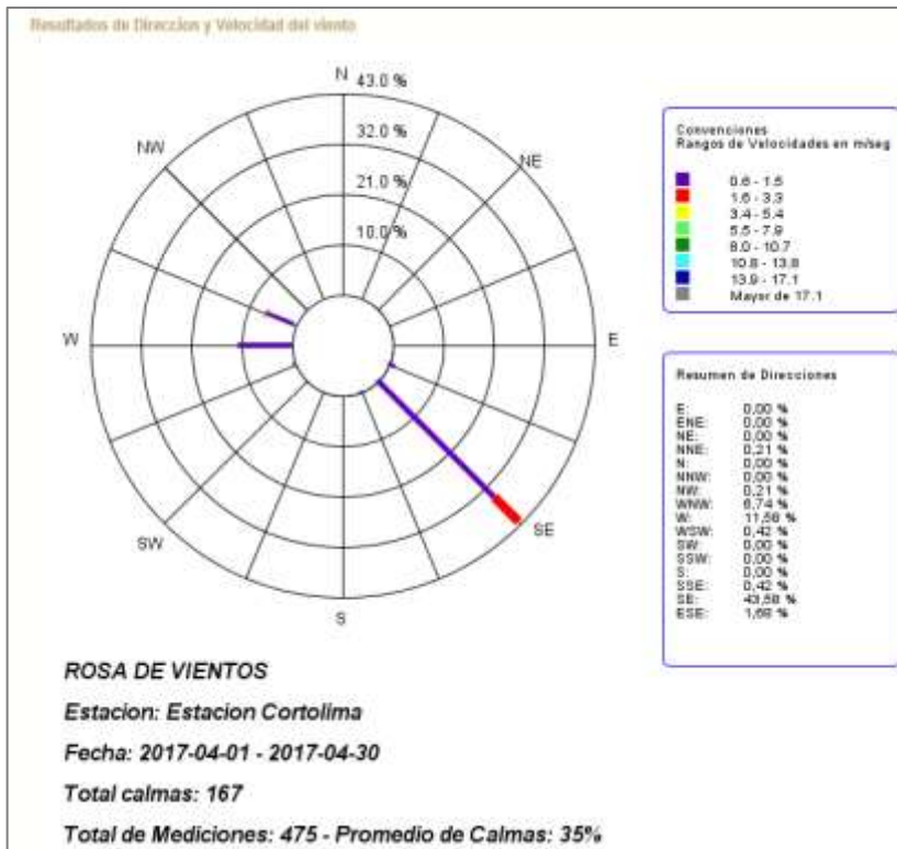
Gráfico3. Rosa de vientos Estación Cortolima Abril 2017.
