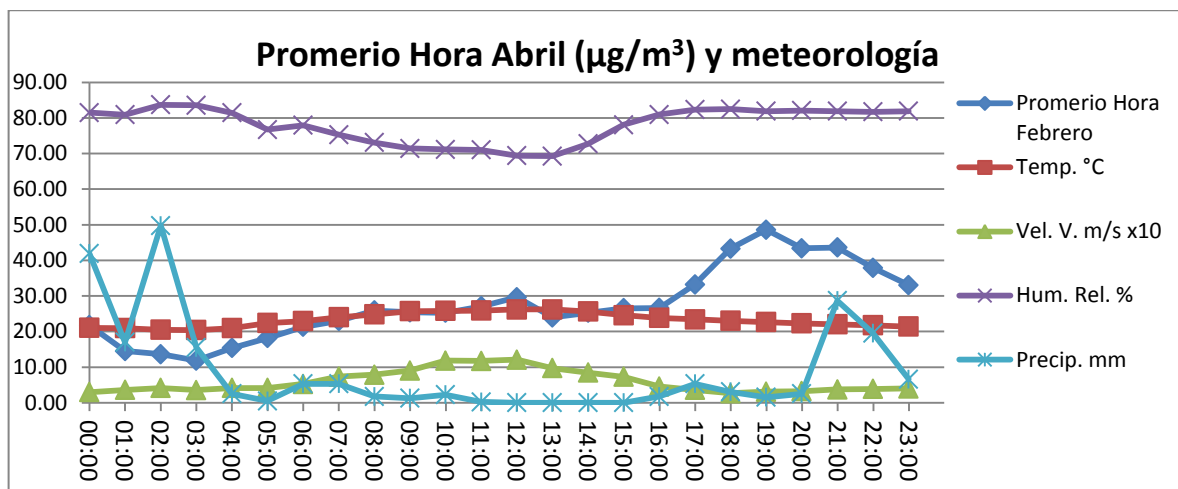
Gráfico 4. Concentraciones promedio por hora PM 10 y data meteorológica Estación Cortolima Abril 2017.
