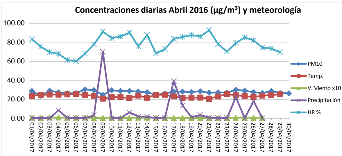
Gráfico 1. Concentraciones PM 10 y data meteorológica diaria Estación Cortolima Abril 2017.
