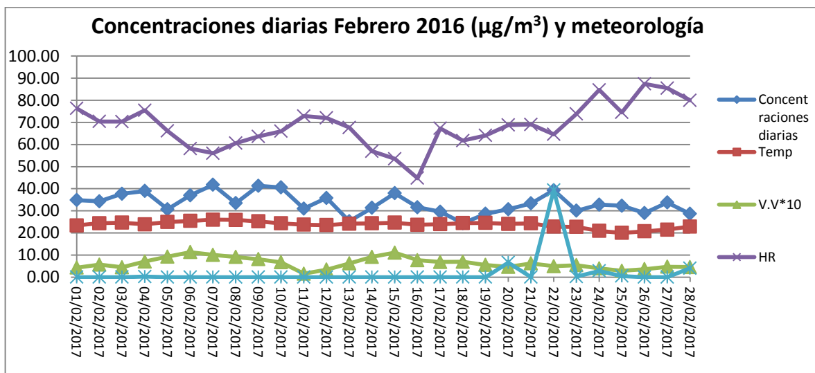
Gráfico 7. Concentraciones PM 10 y data meteorológica diaria Estación Cortolima febrero 2017.
