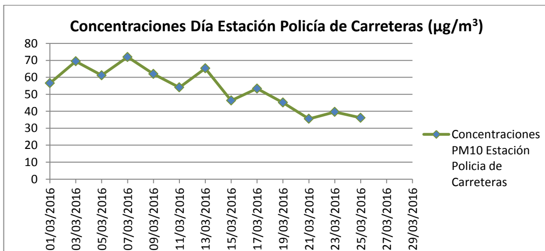
Gráfico 11. Concentraciones diarias PM 10 Estación Policía de Carreteras febrero de 2017.
