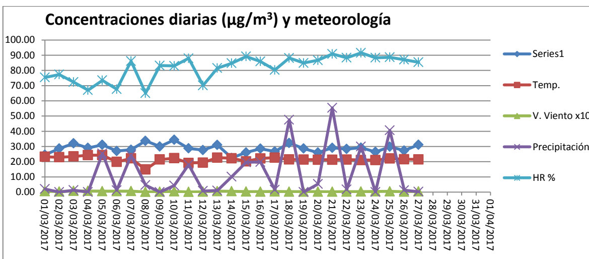
Gráfico 13. Concentraciones \text{PM}_{10} y data meteorológica diaria Estación Cortolima marzo 2017.
