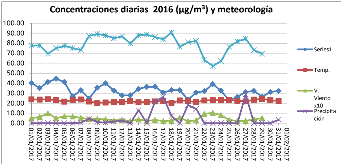
Gráfico 1. Concentraciones \text{PM}_{10} y data meteorológica diaria Estación Cortolima Enero 2017.
