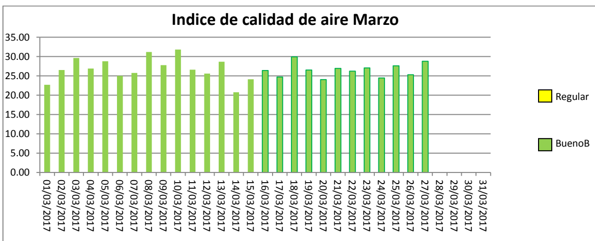
Gráfico 14. Índices de calidad de aire Estación Cortolima marzo 2017.
