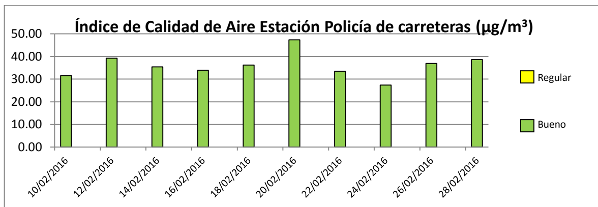
Gráfico 6. Índice de Calidad de Aire Estación Policía de Carreteras Enero 2017.
