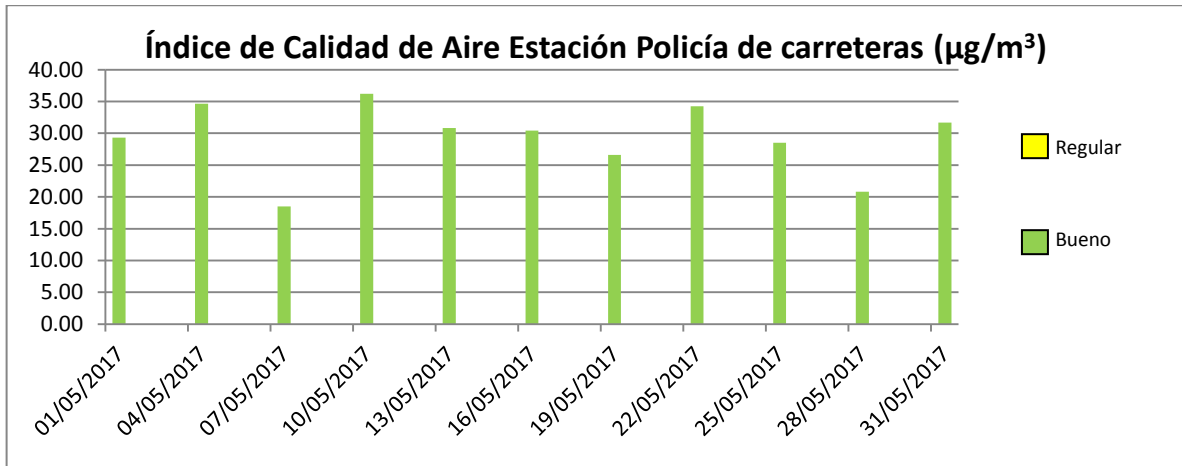
Gráfico 6. Índice de Calidad de Aire Estación Policía de Carreteras Mayo 2017.
