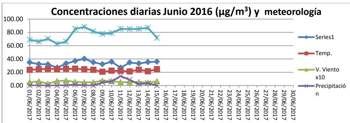
Gráfico 1. Concentraciones PM 10 y data meteorológica diaria Estación Cortolima Junio 2017.
