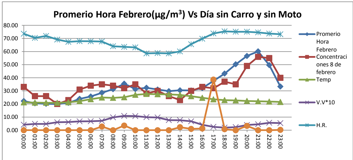
Gráfico 10. Concentraciones promedio por hora PM 10 y data meteorológica Estación Cortolima febrero de 2017.
