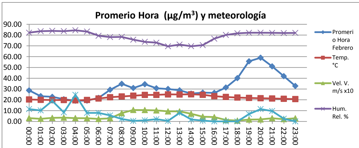
Gráfico 4. Concentraciones promedio por hora PM 10 y data meteorológica Estación Cortolima Enero 2017.
