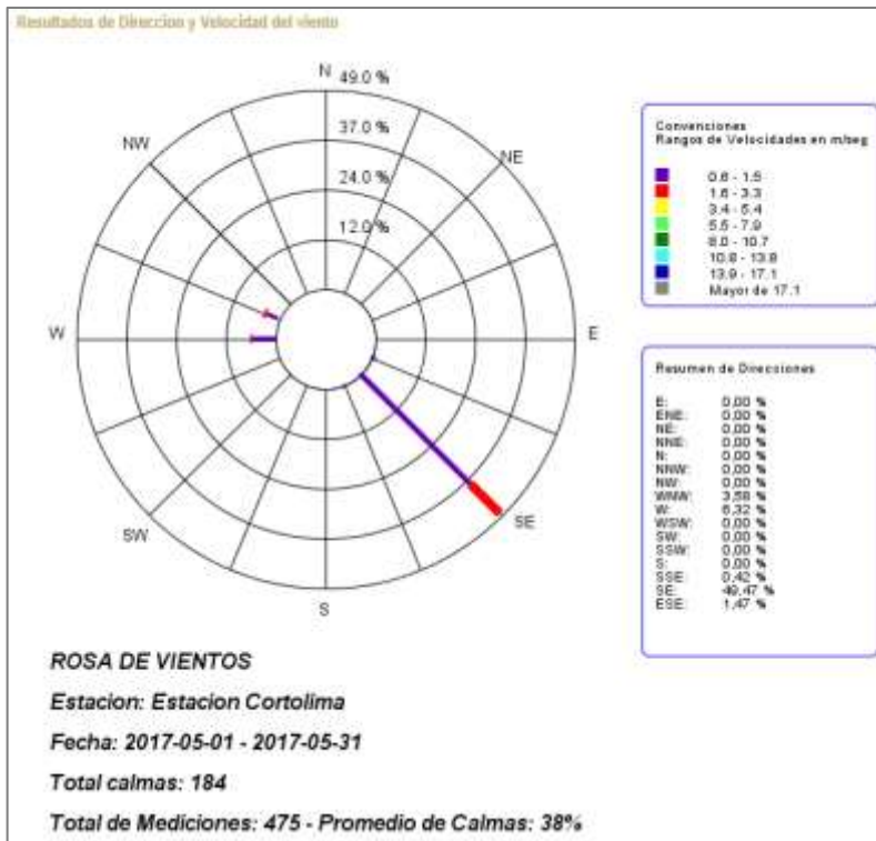
Gráfico3. Rosa de vientos Estación Cortolima Mayo 2017.
