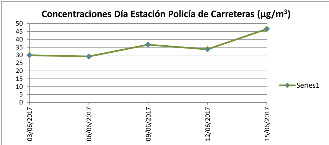
Gráfico 5. Concentraciones diarias PM 10 Estación Policía de Carreteras Junio 2017.
