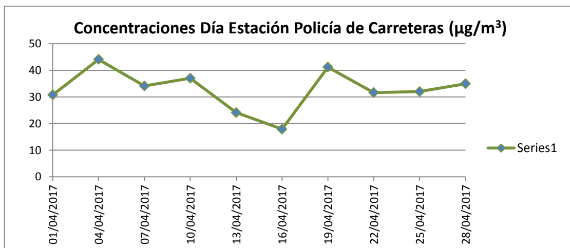
Gráfico 5. Concentraciones diarias PM 10 Estación Policía de Carreteras Abril 2017.
