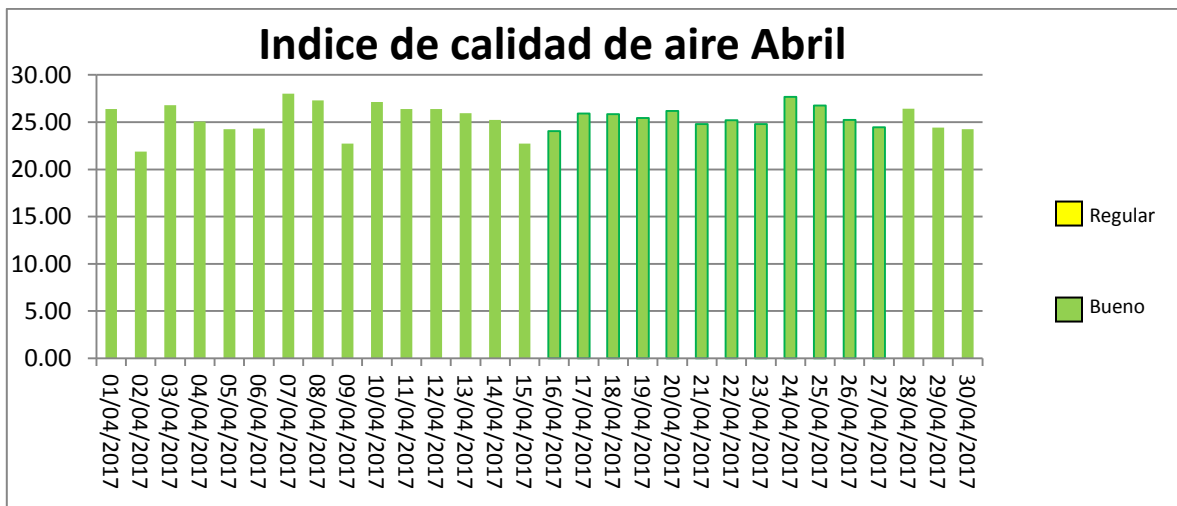
Gráfico 2. Índices de calidad de aire Estación Cortolima Abril 2017.
