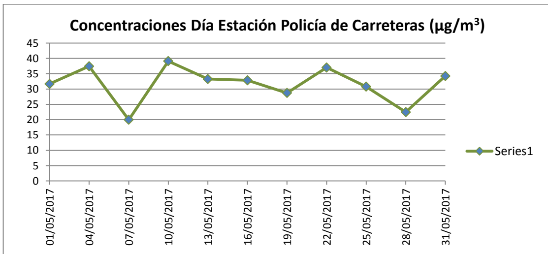
Gráfico 5. Concentraciones diarias PM_{10} Estación Policía de Carreteras Mayo 2017.
