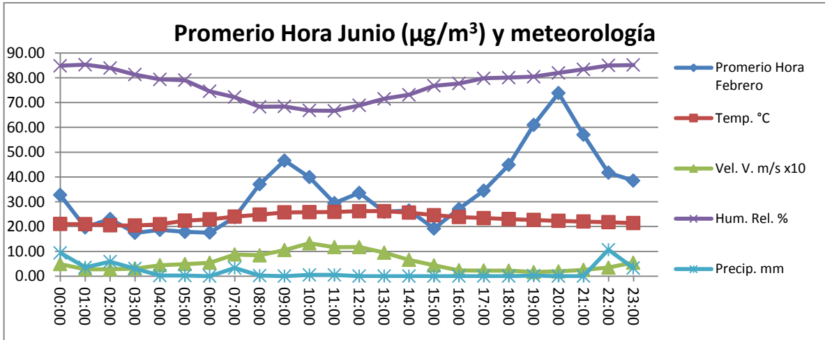
Gráfico 4. Concentraciones promedio por hora PM 10 y data meteorológica Estación Cortolima Junio 2017.
