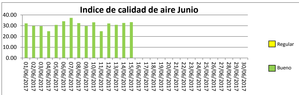
Gráfico 2. Índices de calidad de aire Estación Cortolima Junio 2017.
