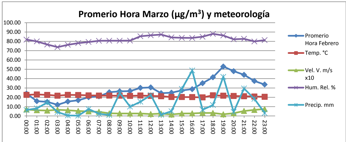
Gráfico 16. Concentraciones promedio por hora PM 10 y data meteorológica Estación Cortolima marzo 2017.
