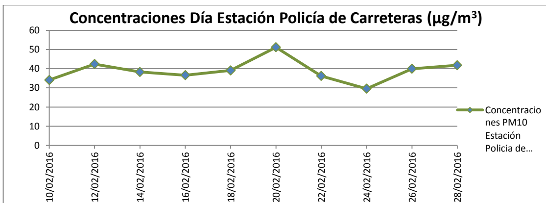
Gráfico 5. Concentraciones diarias PM 10 Estación Policía de Carreteras Enero 2016.
