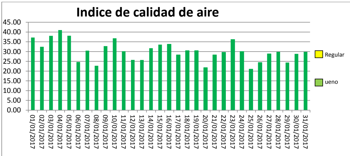
Gráfico 2. Índices de calidad de aire Estación Cortolima Enero 2017.
