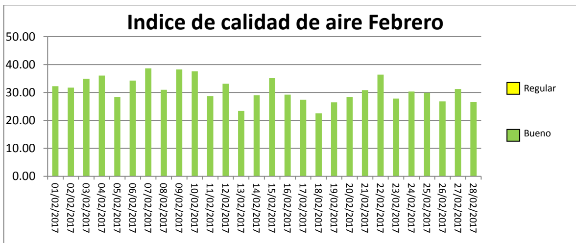
Gráfico 8. Índices de calidad de aire Estación Cortolima febrero 2017.
