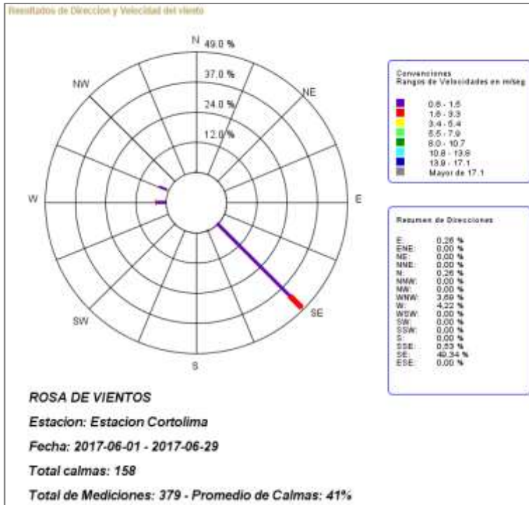
Gráfico3. Rosa de vientos Estación Cortolima Junio 2017.
