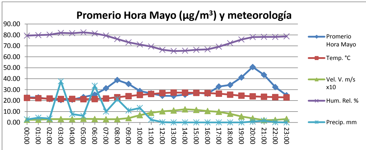
Gráfico 4. Concentraciones promedio por hora PM_{10} y data meteorológica Estación Cortolima Mayo 2017.
